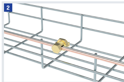
2 Garantizar una adecuada continuidad eléctrica y una adecuada puesta a tierra para disipar corrientes y evitar acumulación de potencial eléctrico.
