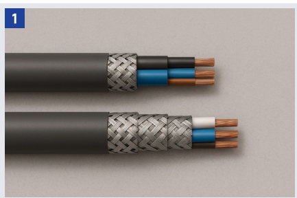
1 Utilizar cables blindados
