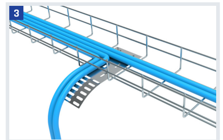
3 Los cables deben cruzarse a 90° (ángulo recto). Evitar cruces perpendiculares entre cables de potencia y datos.
