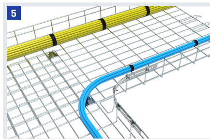
5 Disposición adecuada de los cables en la bandeja.
