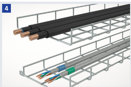
4 Separar cables de datos y energía. Usar bandejas independientes para cada tipo de cableado.
