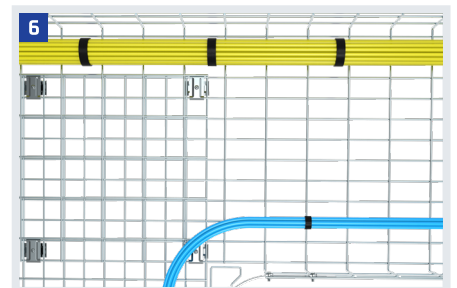
6 La distancia entre los cables de alimentación y de control debe ser al menos 5 veces el radio del cable de alimentación más grande.
